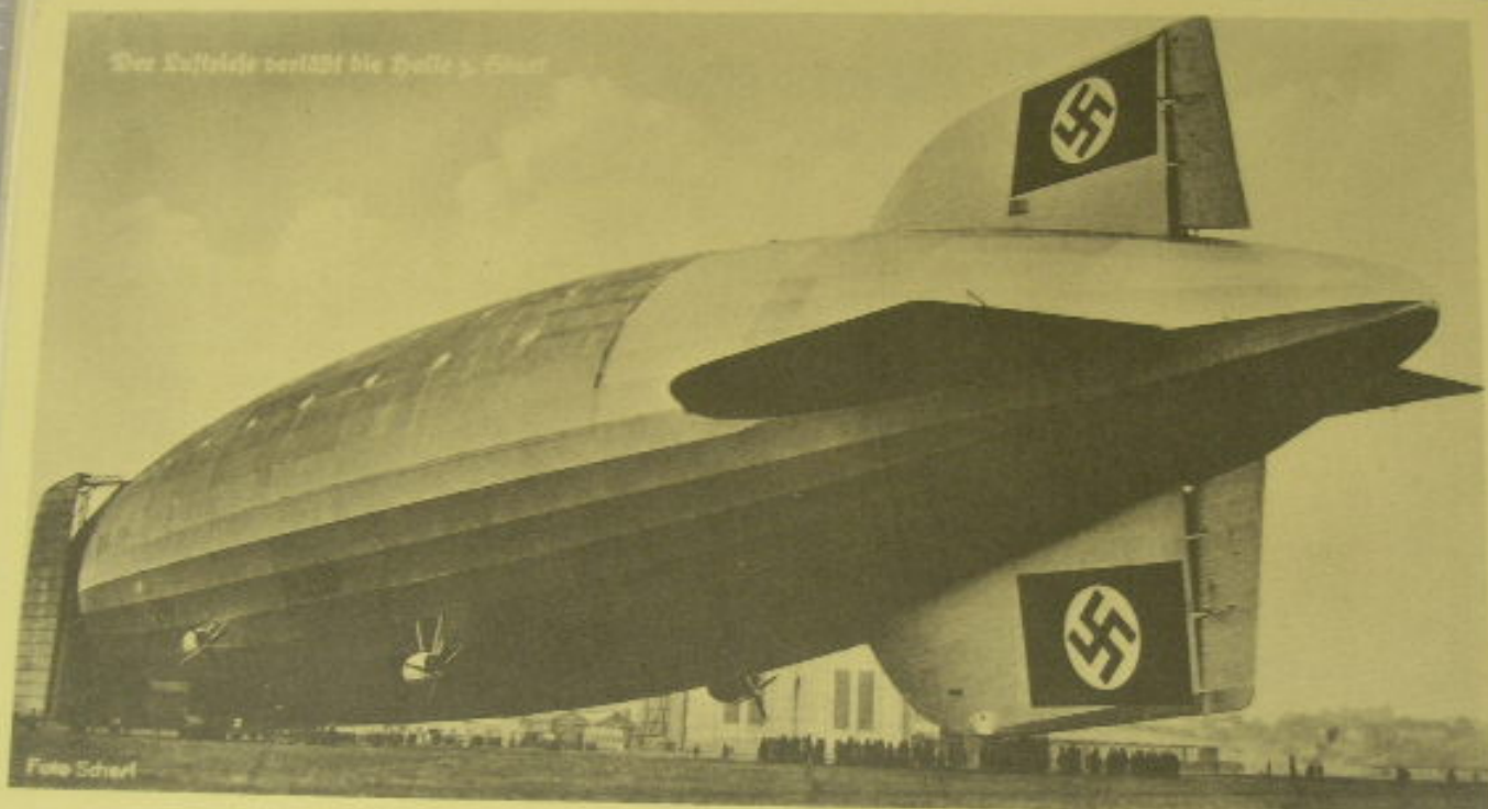
Der Luftschiff verlässt die Halle v. Schierl Foto Schierl Das neue deutsche Zeppelin-Luftschiff „Hindenburg“ L. Z. 129 Das größte Luftschiff der Welt. Länge 248 m. Höhe 44,7 m, größter Durchmesser 41,2 m. Vortriebsmaschinen: 4 Mercedes-Benz Dieselmotore von je 1100 PS Geschwindigkeit von etwa 130 Stdkm.
