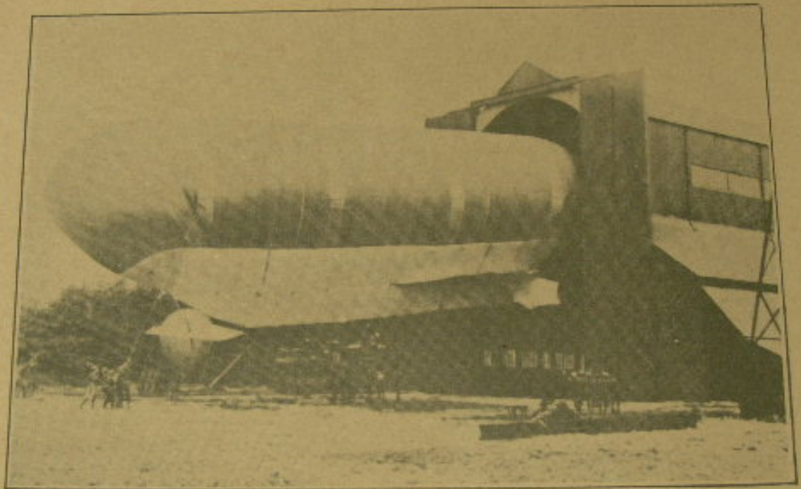
54 • DIRIGIBLE N o II
